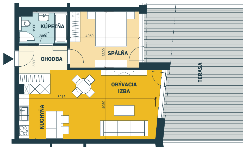
schéma podlažia
