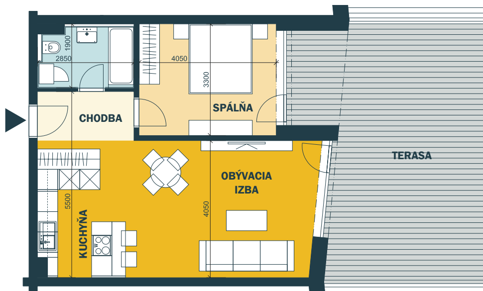
schéma podlažia
